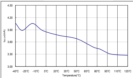
图 9. 工作电流
