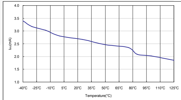
图 10. 从引脚 HV 可提供电流
