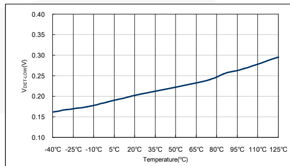
图 12. 箝位电压下限
