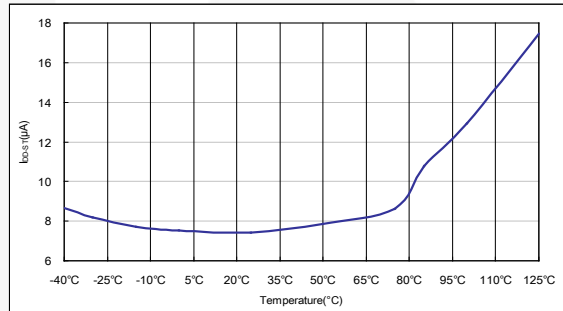
图 8. 启动电流
