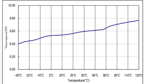
图 6. PWM 关断阈值电压
